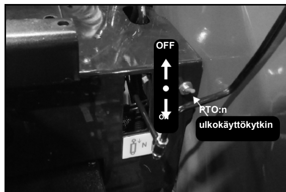
Kuva a: Mallin 20 kytkin
