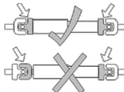
Nivelakselin nivelet
