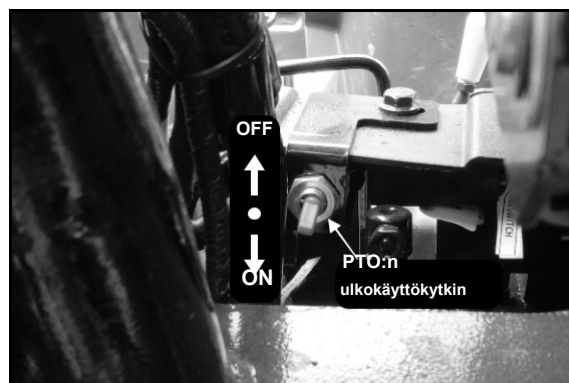
Kuva b: Mallin 26 kytkin
