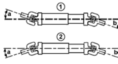
Nivelakselin nivelet
